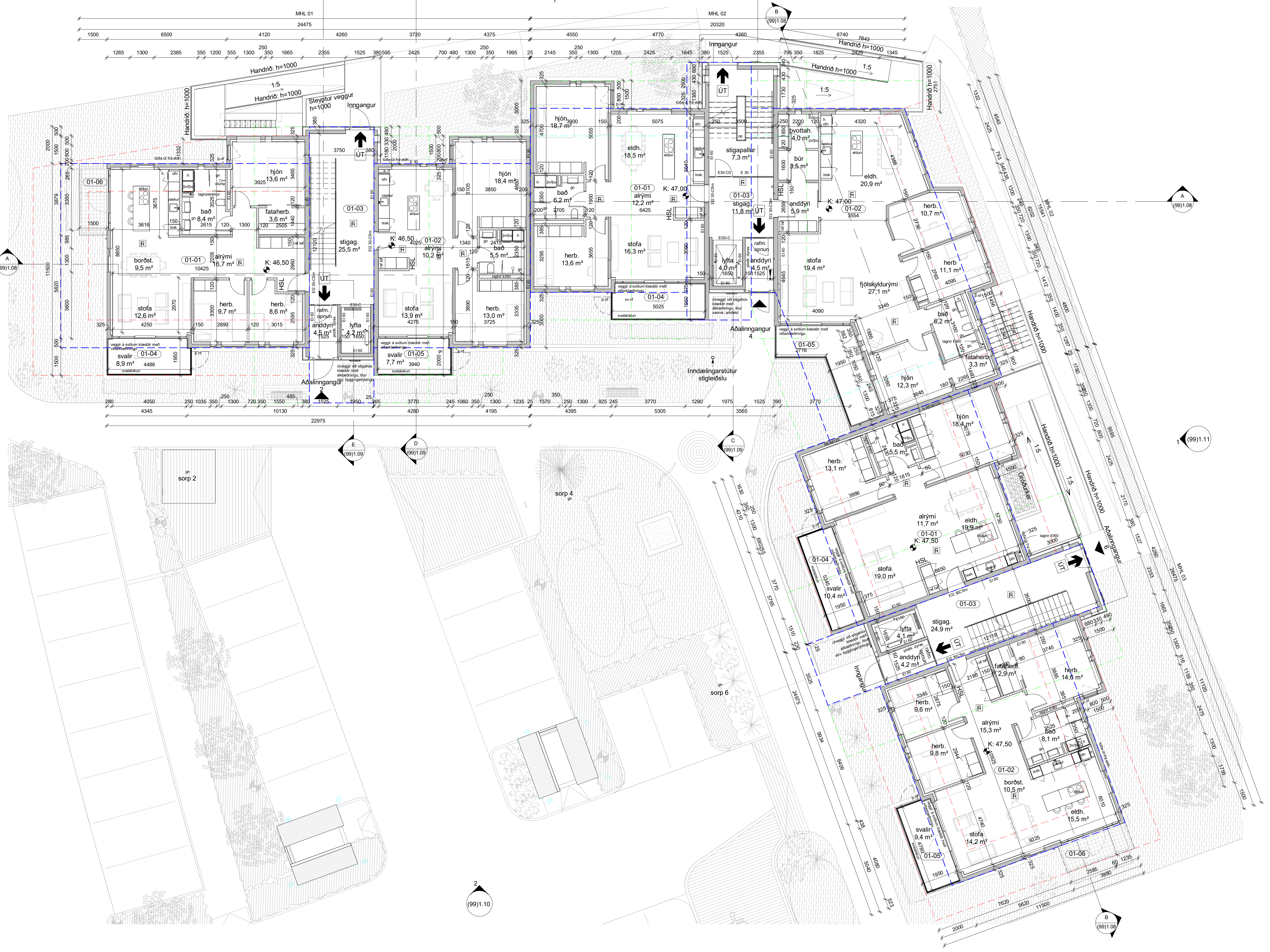
1 Grunnmynd- 1. hæð 1: 100
